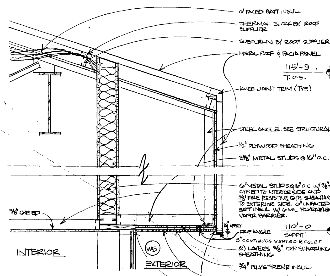
6 SOFFIT DETAIL A3.3 SCALE: 3/4" = 1'-0"
