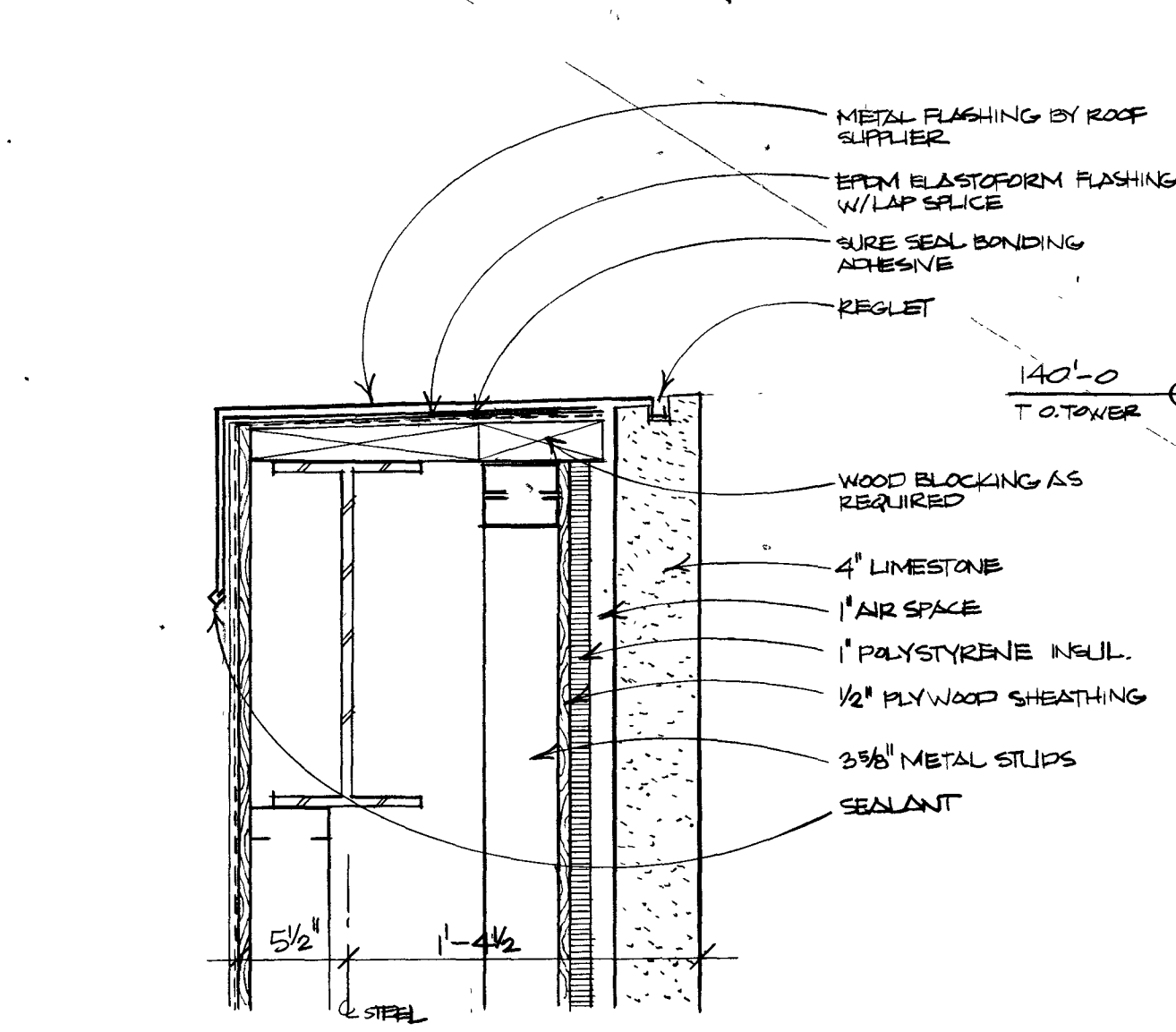
5 PARAPET DETAIL A3.3 SCALE: 1/2" = 1'-0"
