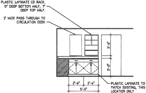
8 CASEWORK ELEVATION SCALE: 1/4" = 1'-0" AV WORK/OFFICES 119
