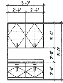
9 CASEWORK ELEVATION SCALE: 1/4" = 1'-0" AV WORK/OFFICES 119
